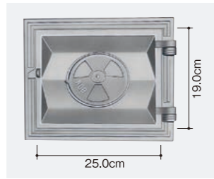
二宮式焚口8号(薄)
