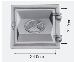
二宮式焚口8号(厚)
