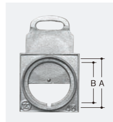
差入式煙突受 (旧スレート煙突対応型)
