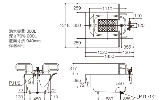
足が入り込みやすい斜め形状のエプロン
