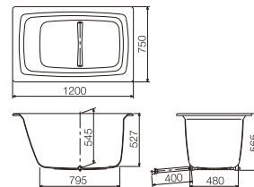
DH-120 L1,200×D750×H565(深さ545)mm 満水容量 250L / 両排水 / 排水パイプ・風呂底付 ¥234,000 (税込 ¥257,400)
