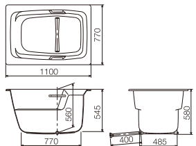
RD-110 L1,100×D770×H580(深さ560)mm 満水容量 250L / 両排水 / 排水パイプ・風呂底付 ¥244,000 (税込 ¥268,400)
