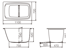
DH-110 L1,100×D720×H557(深さ540)mm 満水容量 240L / 両排水 / 排水パイプ・風呂底付 ¥215,000 (税込 ¥236,500)
