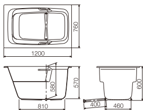
RD-120 L1,200×D760×H600(深さ580)mm 満水容量 280L / 両排水 / 排水パイプ・風呂底付 ¥283,000 (税込 ¥311,300)
