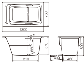
RD-130 L1,300×D760×H600(深さ580)mm 満水容量 285L / 両排水 / 排水パイプ・風呂底付 ¥316,000 (税込 ¥347,600)
