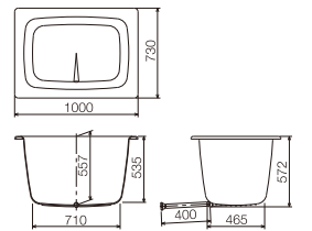
DH-100 L1,000×D730×H572(深さ557)mm 満水容量 220L / 両排水 / 排水パイプ・風呂底付 ¥205,000 (税込 ¥225,500)
