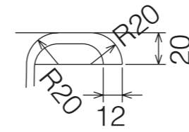
フチ部詳細(4方R)
