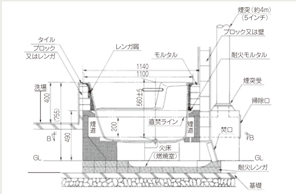
築炉施工図 (RD-1177の例)
